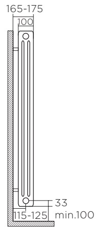
SEITENANSICHT
