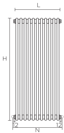
VORDERANSICHT
