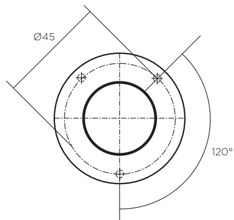
DETAIL BASISPLATTE (Befestigungspunkt)
